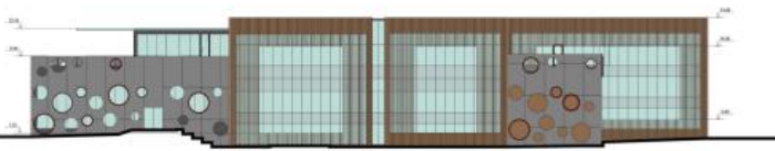
PIETŲ FASADAS, M 1:200
