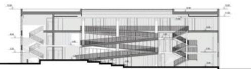
PĖJŪVIS 2-2, M 1:200
