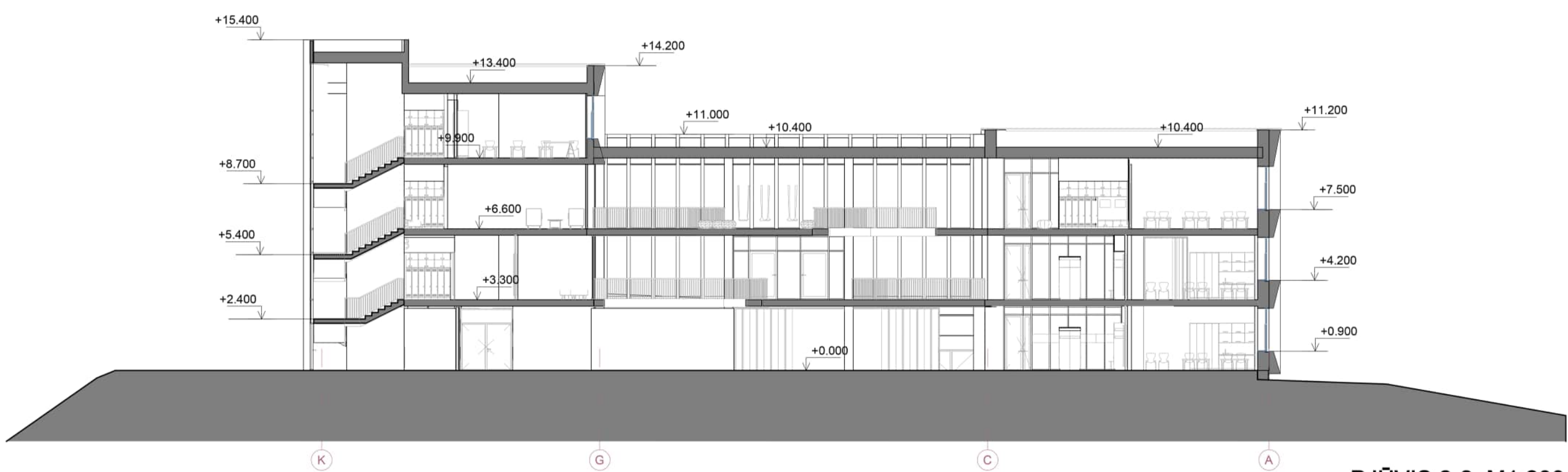
PJŪVIS 2-2, M1:200
