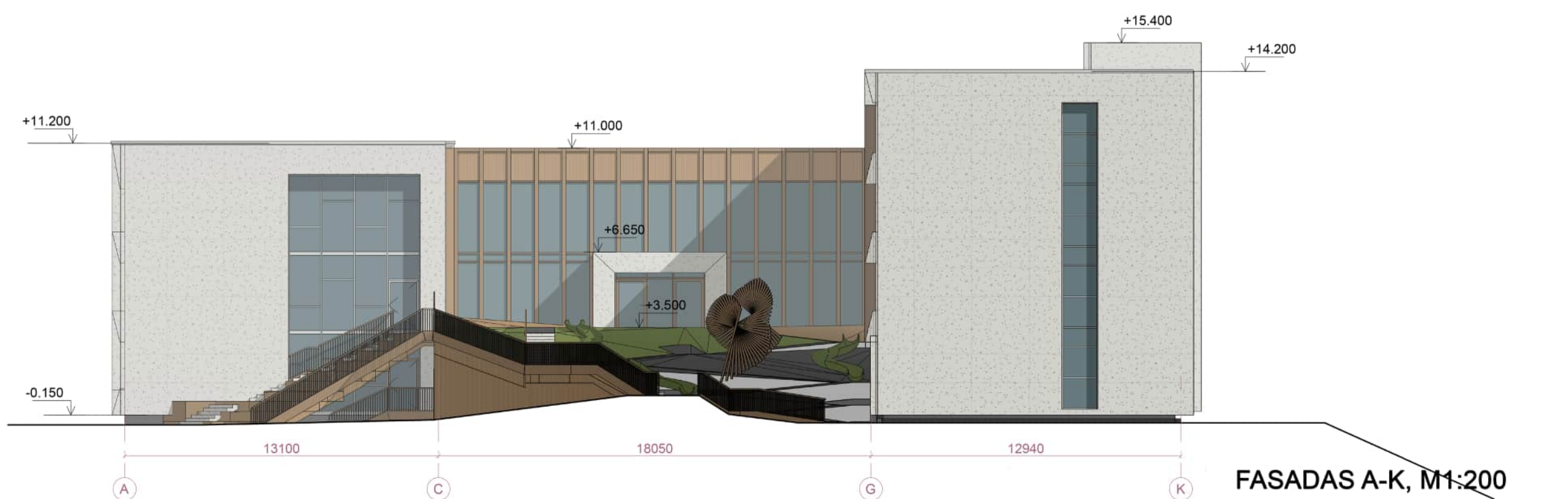
FASADAS A-K, M1:200
