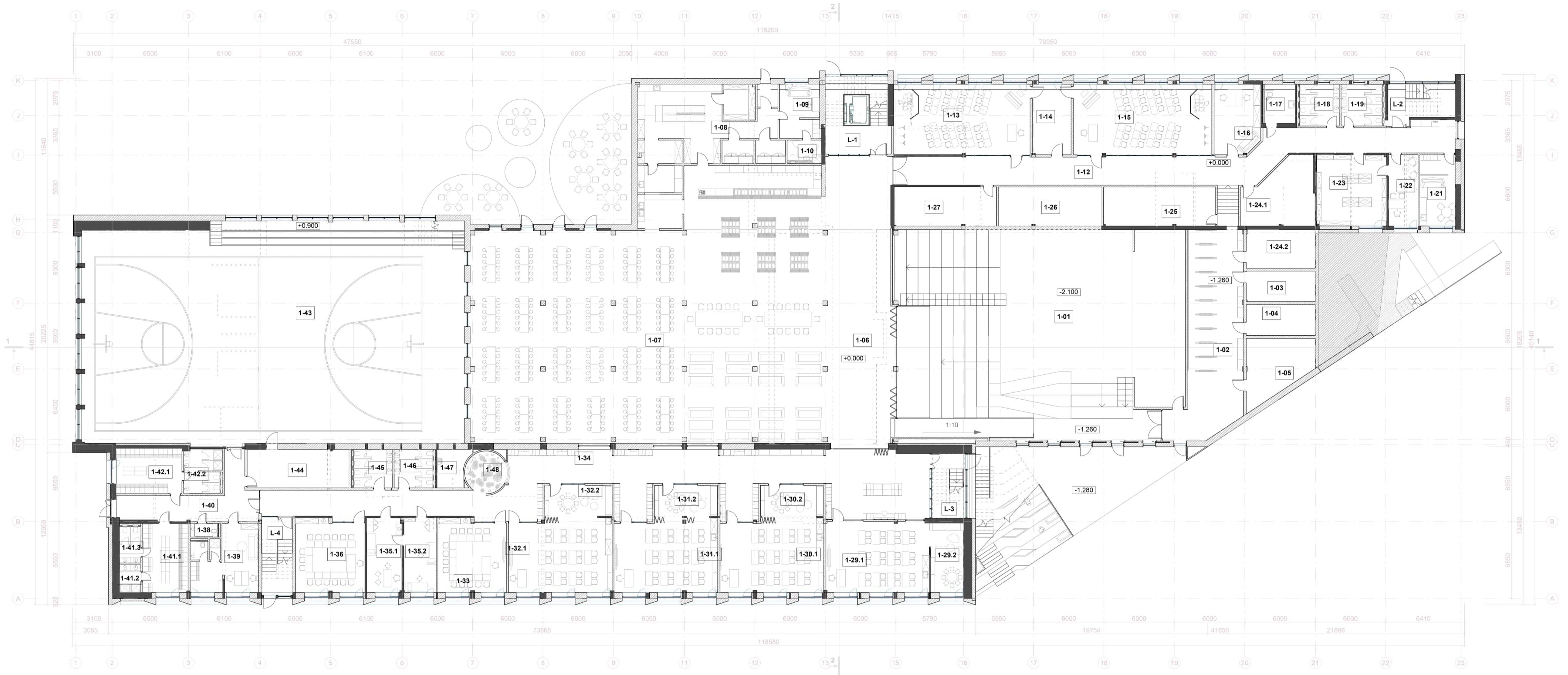
PIRMO AUKŠTO PLANAS, M 1 : 200
