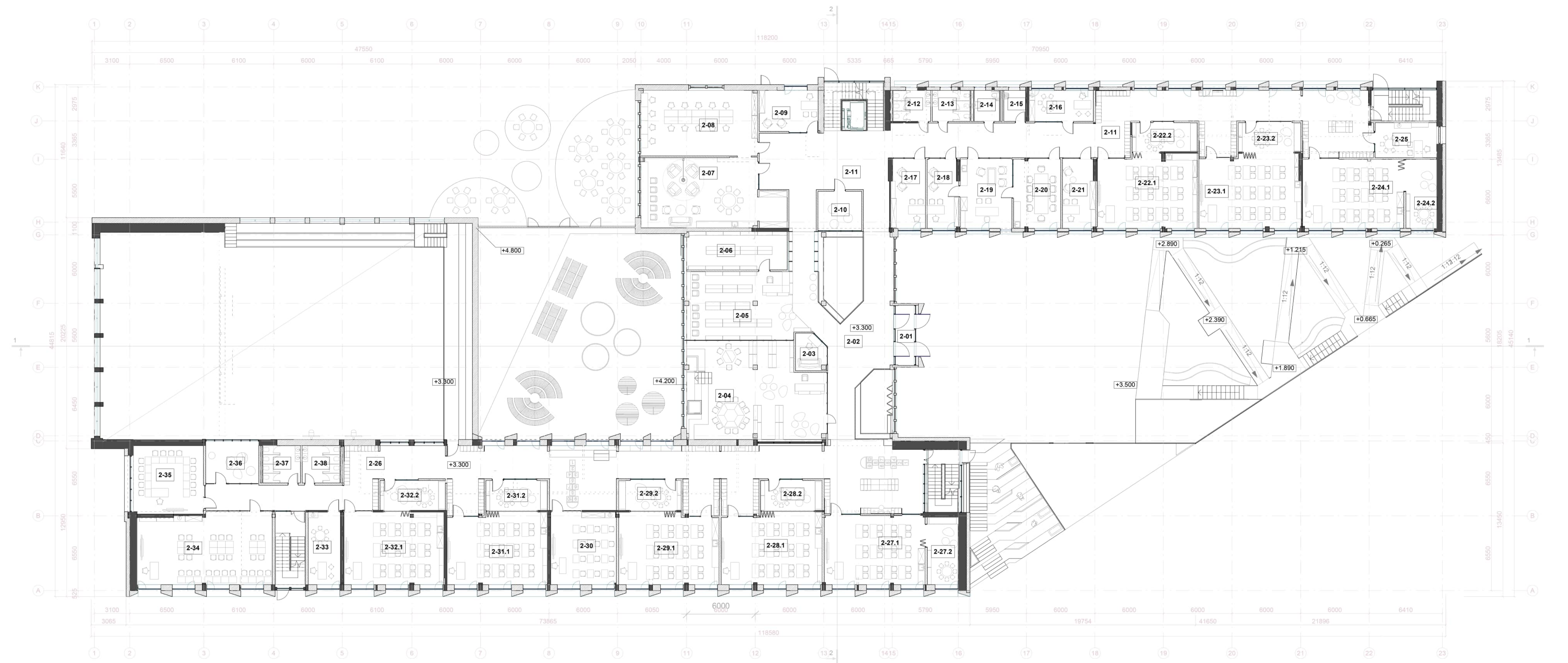
ANTRO AUKŠTO PLANAS, M1:200
