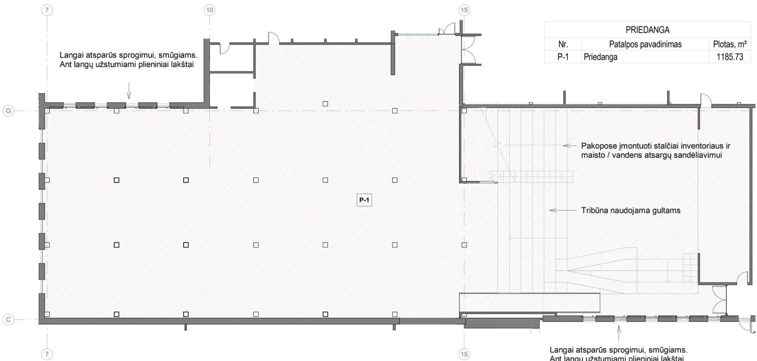
PIRIEDANGOS PLANAS, M 1 : 200
