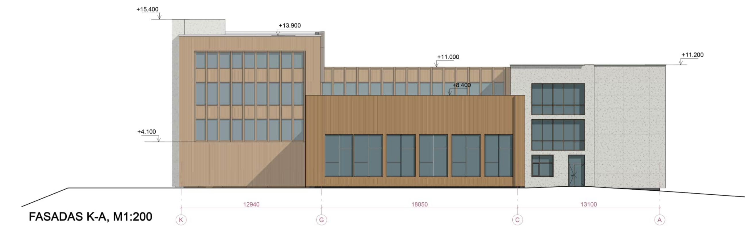
FASADAS K-A, M1:200
